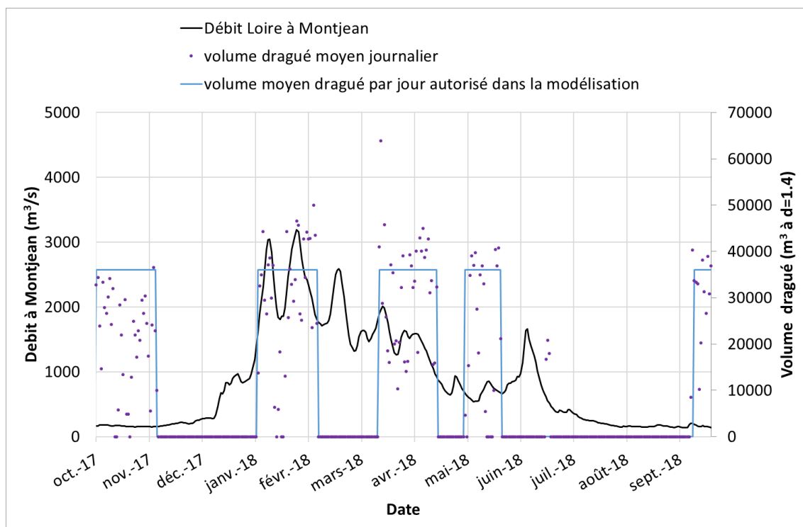
Figure 12 : Périodes de dragages modélisées sur l'année hydrologique 2017-2018
