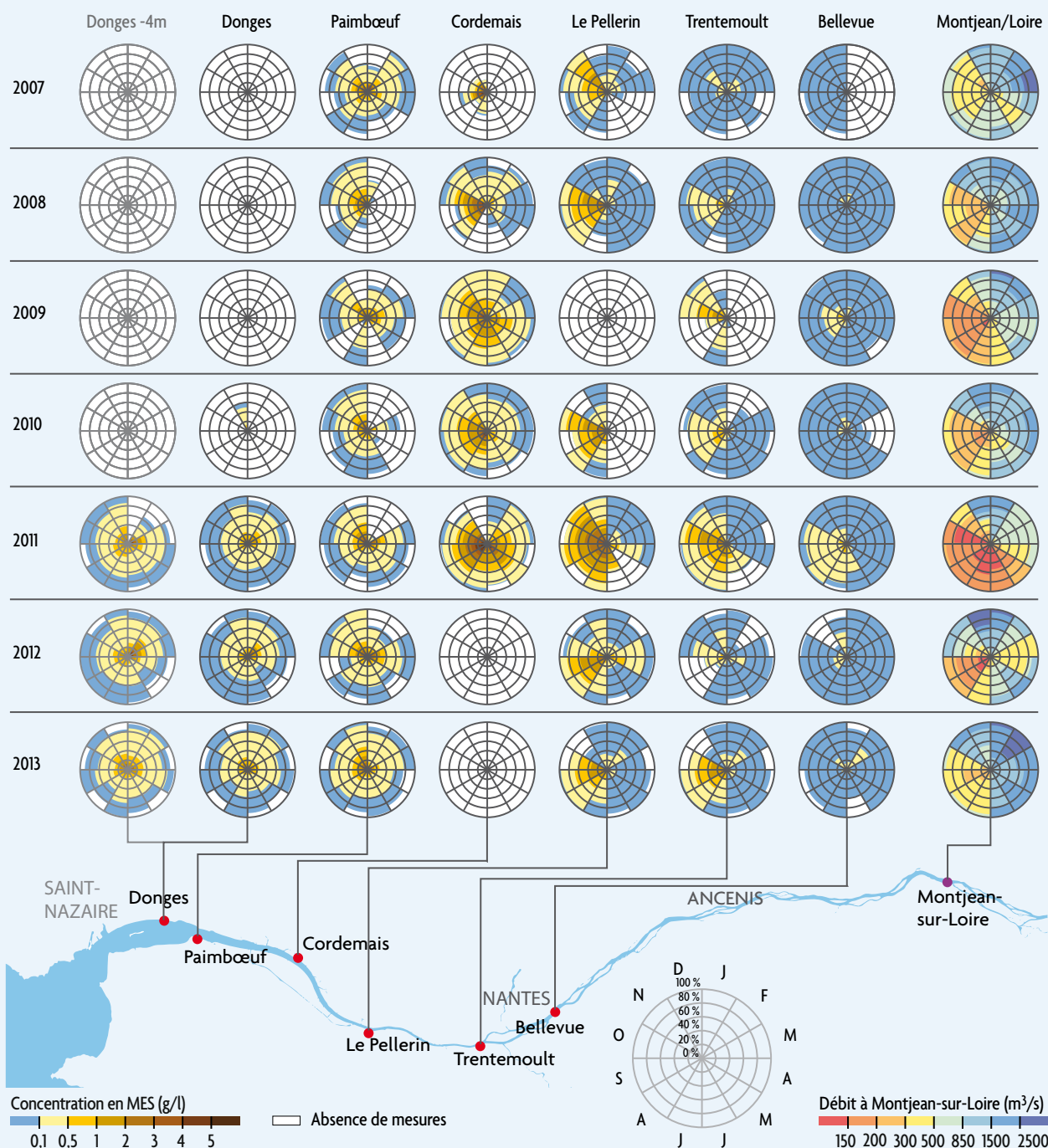
Distribution mensuelle de la concentration en MES au niveau des stations SYVEL et du débit à Montjean-sur-Loire, de 2007 à 2013
