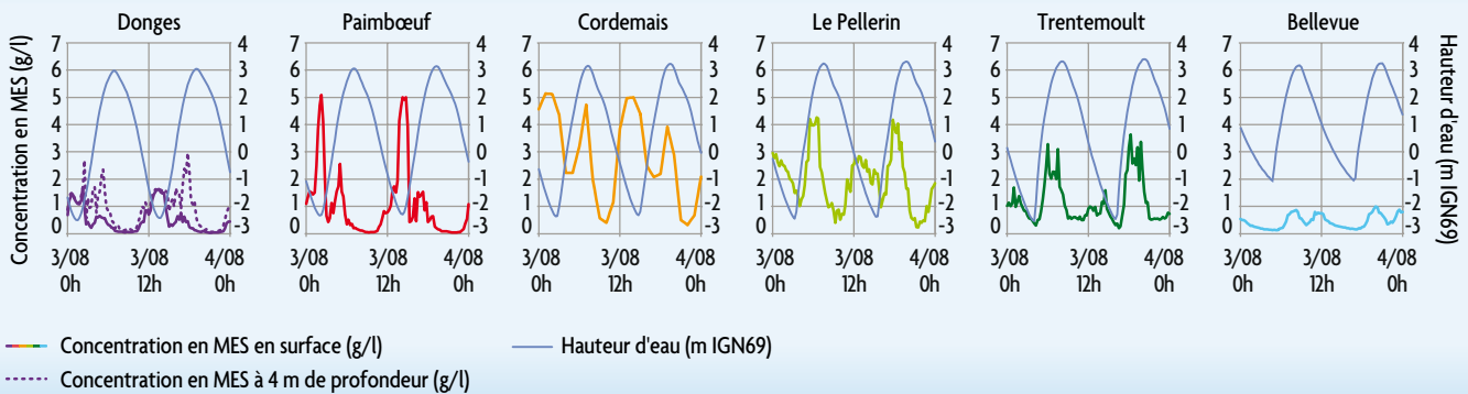
Evolution des concentrations en MES au cours des marées du 3 août 2011 (débit = 149 m 3 /s, coeff. 101-98)
