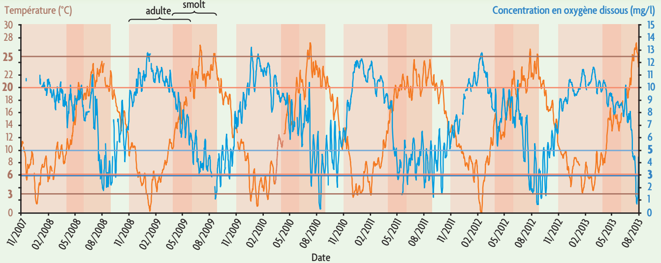
Variations quotidiennes des paramètres température et oxygène dissous dans l'estuaire de la Loire, et influence sur le saumon
