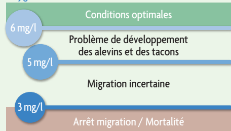
Durée (en nombre de jours) de la période la plus longue sous les seuils d'oxygène dissous dans l'eau
