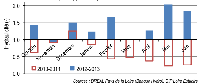
Hydraulicité mensuelle à Montjean-sur-Loire, par rapport à la période 1863-2013
