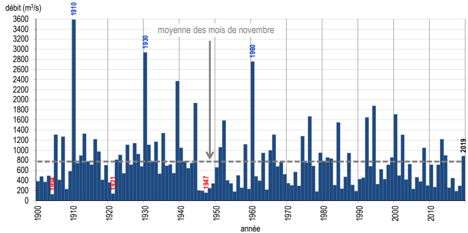
Extraction du débit moyen du mois de novembre à la station de Montjean-sur-Loire, depuis 1900
