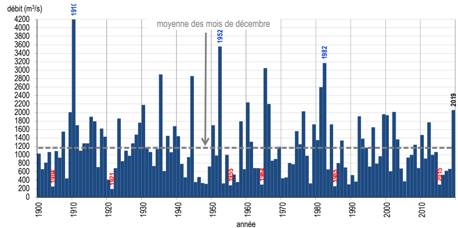
Extraction du débit moyen du mois de décembre à la station de Montjean-sur-Loire, depuis 1900
