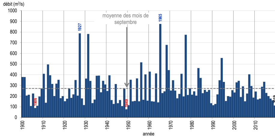
Extraction du débit moyen du mois de septembre à la station de Montjean-sur-Loire, depuis 1900
