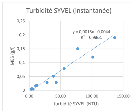
Figure 13 : Concentration en MES (g/l) en fonction de la turbidité instantanée (NTU) mesurée par la sonde SYVEL, sur la station de la Pierre Percée
