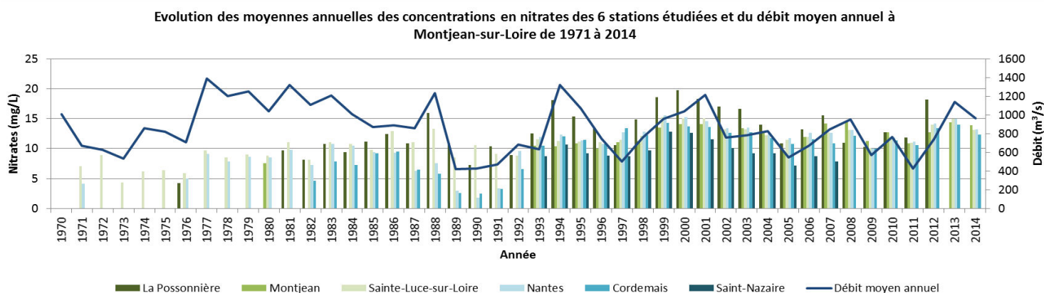
Figure 5 : Synthèse des moyennes annuelles des concentrations en nitrates des 6 stations étudiées et du débit moyen annuel à Montjean-sur-Loire de 1971 à 2014 (sources : AELB, Département44, DDTM44, DREAL Pays de la Loire, GIP Loire Estuaire)
