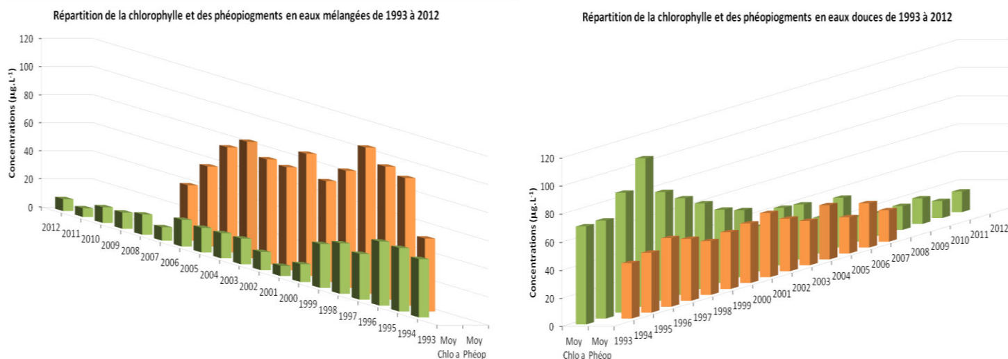
Figure 23 : Synthèse de la répartition de la chlorophylle a et des phéopigments dans les eaux mélangées et les eaux douces entre 1983 et 2012, date à laquelle les données existent pour chacun des six stations étudiées (sources : AELB, Département44, DDTM44, GIP Loire Estuaire)
