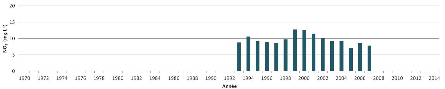
Evolution de la moyenne annuelle des concentrations en nitrates à Saint-Nazaire/Mindin de 1993 à 2007
