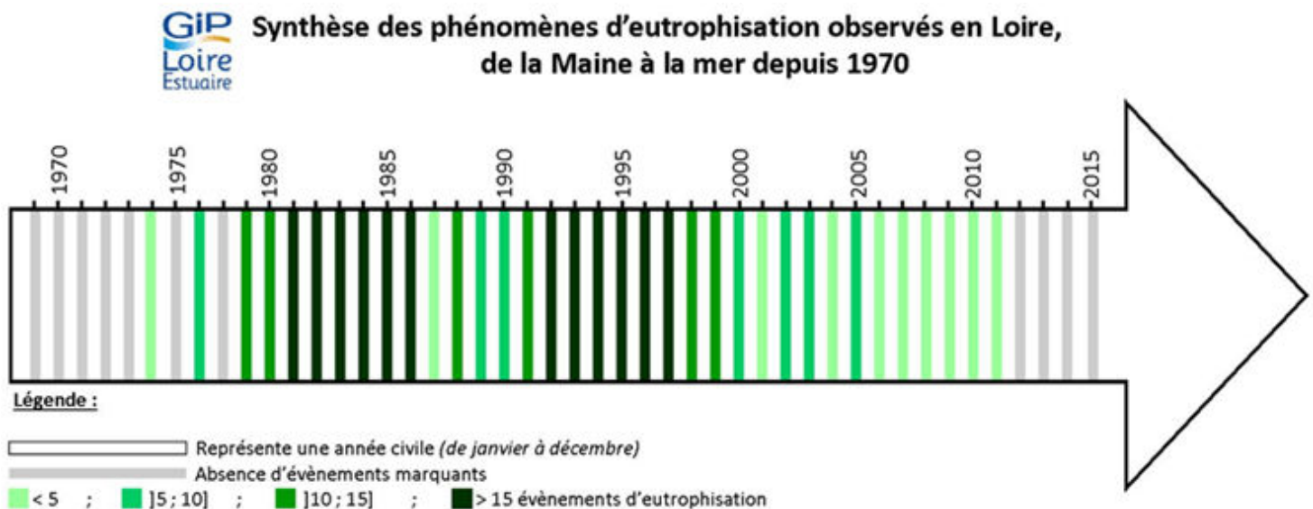
Figure 32 : Synthèse chronologique des évènements d'eutrophisation recensés en Loire, de la Maine à la mer de 1970 à 2014
