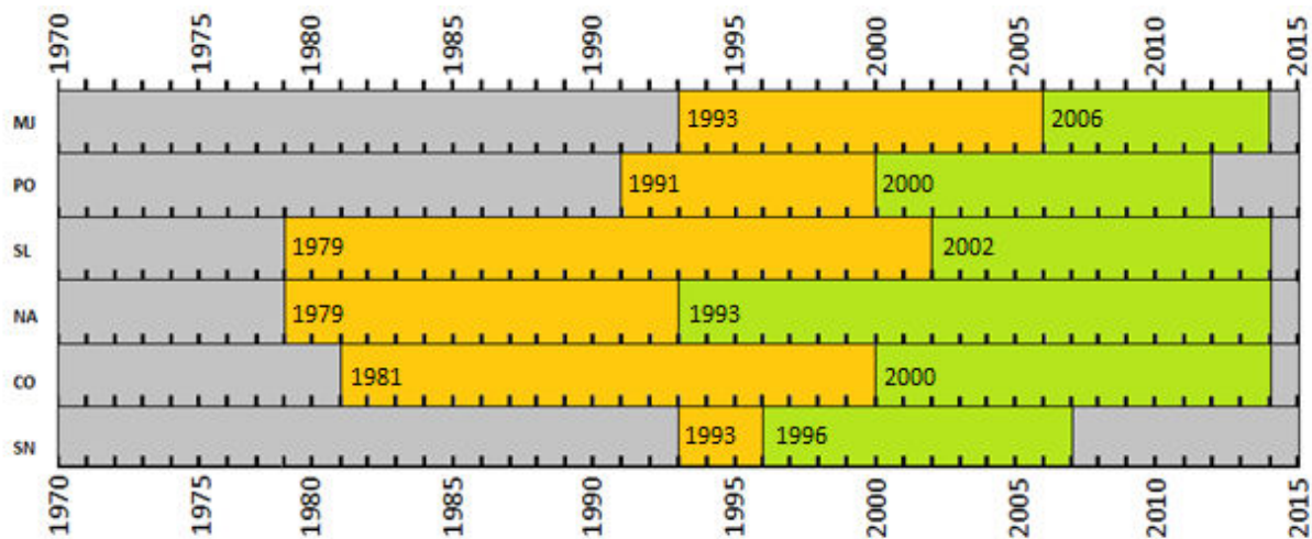
Figure 28 : Schéma présentant le décalage saisonnier des maximums de concentration en chlorophylle a observé dans le temps (Période estivale en orange et printanière en vert ; absence de données en gris)
