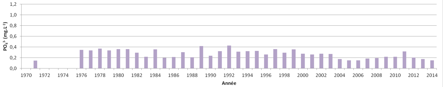
Evolution de la moyenne annuelle des concentrations en phosphates à Nantes/indre de 1971 à 2014
