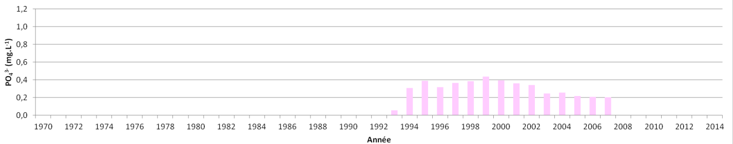
Evolution de la moyenne annuelle des concentrations en phosphates à Saint-Nazaire/Mindin 1993 à 2007
