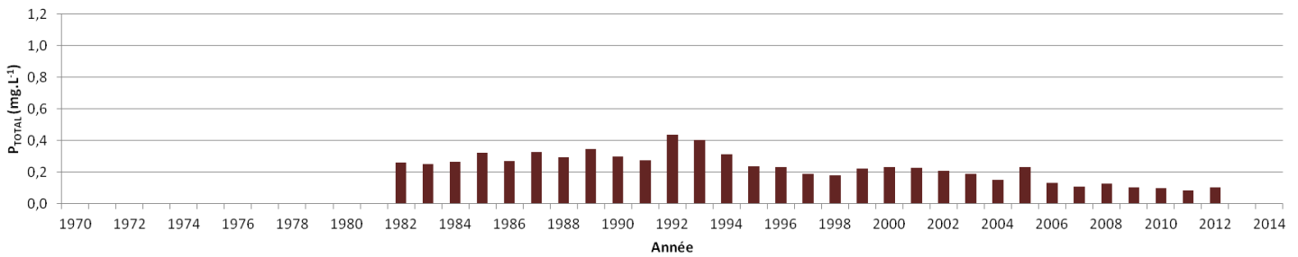
Evolution de la moyenne annuelle des concentrations en phosphore total à La Possonnière de 1982 à 2012
