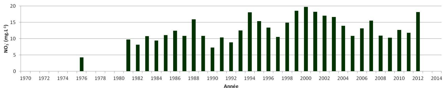
Evolution de la moyenne annuelle des concentrations en nitrates à La Possonnière de 1976 à 2012
