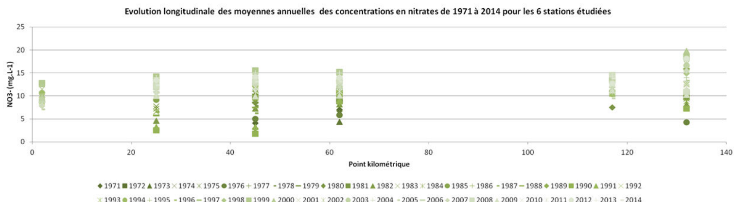
Figure 4: Synthèse de l'évolution longitudinale des moyennes annuelles des concentrations en nitrates de 1971 à 2014 pour les 6 stations étudiées, Points kilométriques : SN (2), CO (25), NA (45), SL (62), MJ (117), PO (132), (sources : AELB, Département 44, DDTM44, GIP Loire Estuaire)
