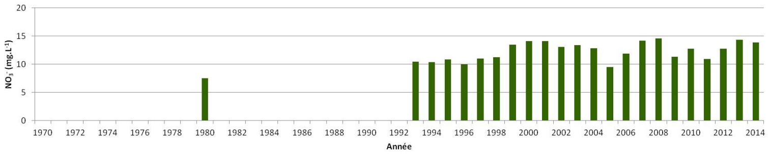
Evolution de la moyenne annuelle des concentrations en nitrates à Sainte-Luce-sur-Loire de 1971 à 2014
