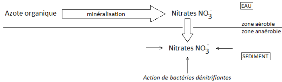
Figure 29 : Schéma de la diffusion des nitrates à l'interface eau/sédiment
