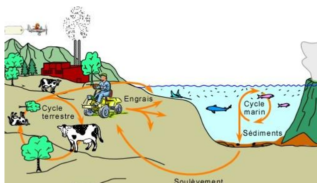
Figure 8 : Cycle terrestre et océanique du phosphore (source : Bourque, 2010)
