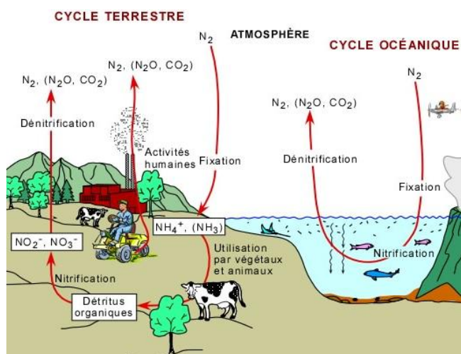
Figure 7 : Cycle terrestre et océanique de l'azote (source : Bourque, 2010)
