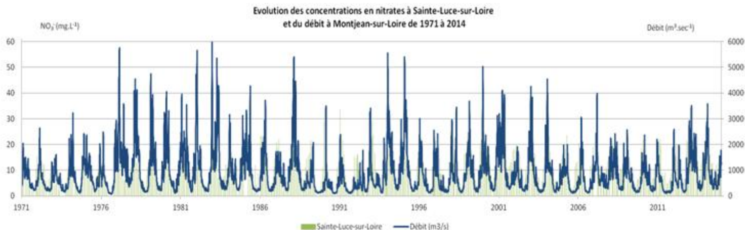
Figure 1 : Graphique de l'évolution des concentrations en nitrates à Sainte-Luce-sur-Loire et du débit à Montjean-sur-Loire de 1971 à 2014 (sources : AELB, Département 44, DDTM44, DREAL Pays de la Loire, GIP Loire Estuaire)
