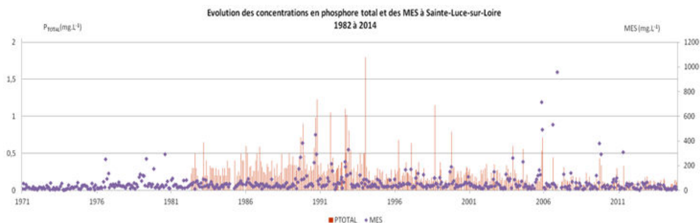
Figure 6 : Graphique de l'évolution des concentrations en phosphore total et des MES à Sainte-Luce-sur-Loire de 1971 à 2014, (sources : AELB, Département44, DDTM44, GIP Loire Estuaire)
