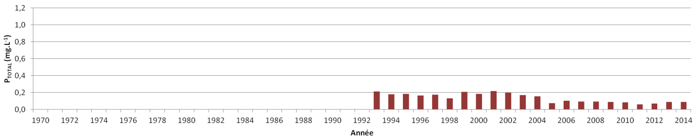
Evolution de la moyenne annuelle des concentrations en phosphore total à Montjean de 1993 à 2014
