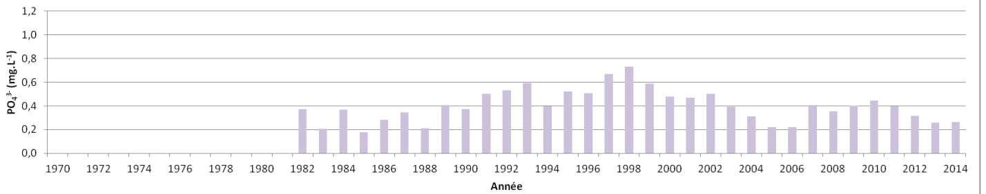
Evolution de la moyenne annuelle des concentrations en phosphates à Cordemais de 1982 à 2014
