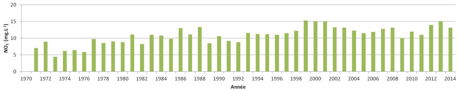
Evolution de la moyenne annuelle des concentrations en nitrates à Nantes/indre de 1971 à 2014
