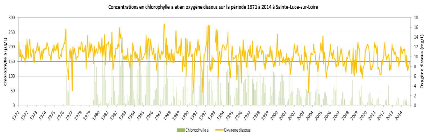
Figure 26 : Graphique de l'évolution de la concentration en chlorophylle a et en oxygène dissous à Sainte-Luce-sur-Loire de 1971 à 2014 (sources : AELB, Département44, DDTM44, GIP Loire Estuaire)
