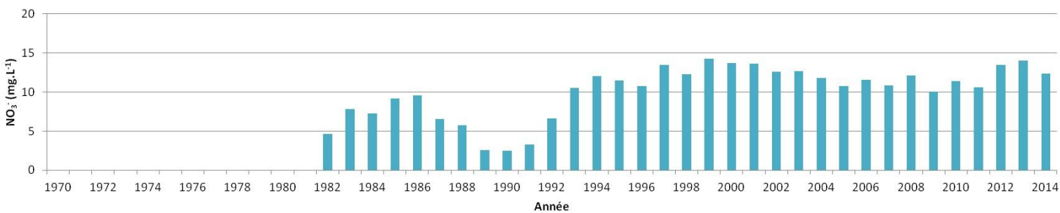
Evolution de la moyenne annuelle des concentrations en nitrates à Cordemais de 1982 à 2014
