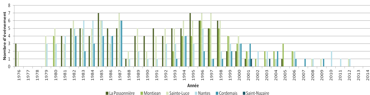
Figure 30 : Graphique de l'évolution du nombre de phénomènes d'eutrophisation en Loire, de la Maine à la mer entre 1976 et 2014 (sources : AELB, Département44, DDTM44, GIP Loire Estuaire)
