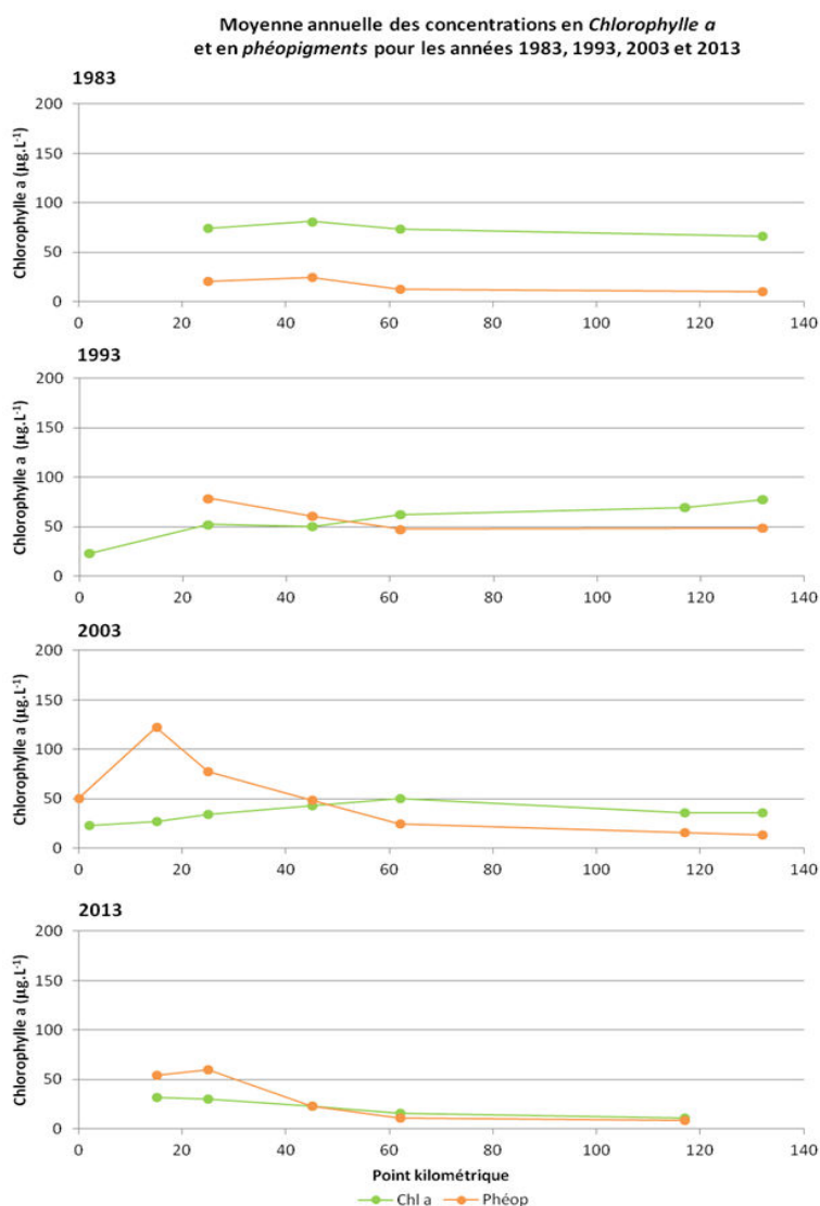
Figure 22 : Synthèse des moyennes annuelles de concentrations en chlorophylle a et en phéopigments pour les années 1983, 1993, 2003 et 2013 (sources : AELB, Département44, DDTM44, GIP Loire Estuaire)
